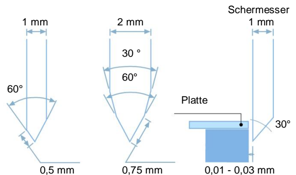
Abb. 3: Saubere Schnittkanten
